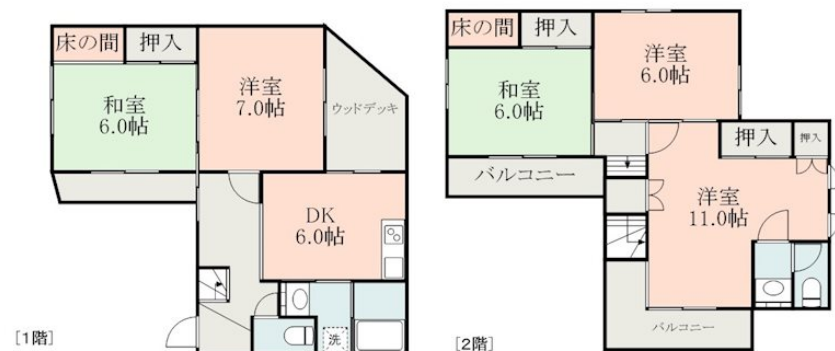
【間取り図】
