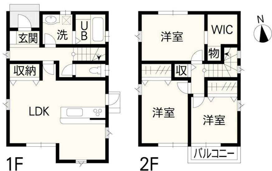
【間取り図】
