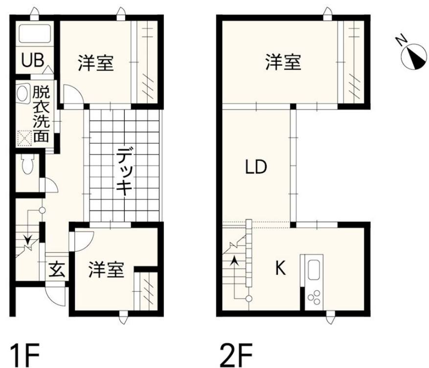
【間取り図】
