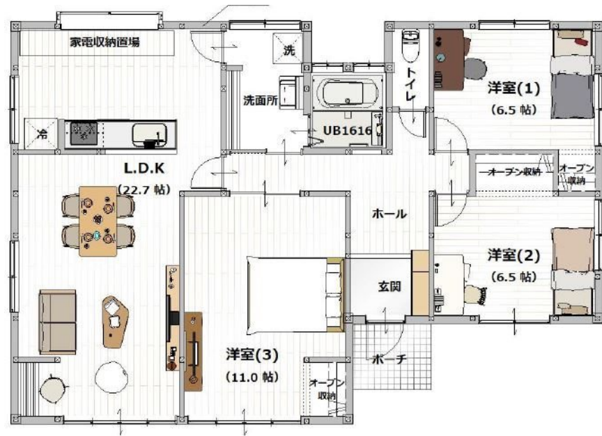
【間取り図】
