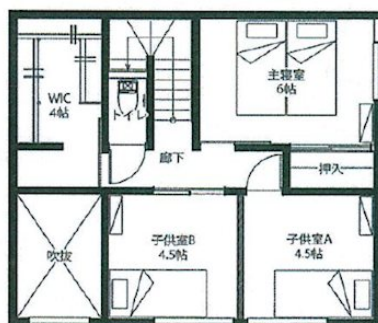
【2階平面図】
