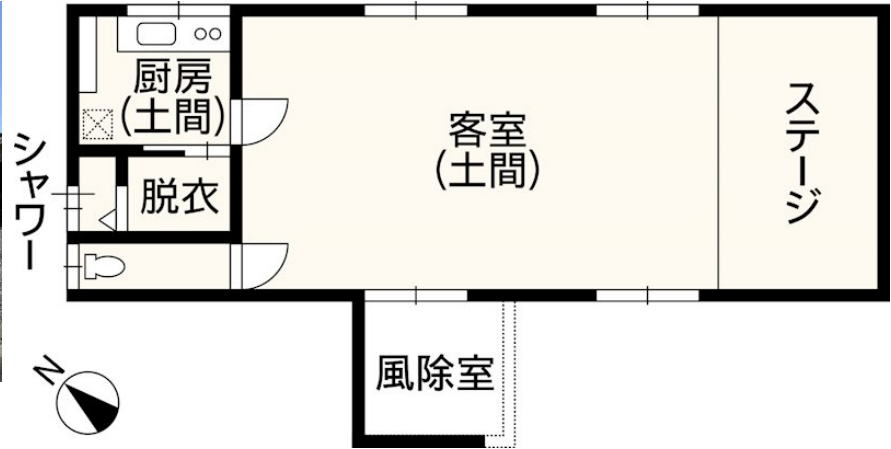
【間取り図】
