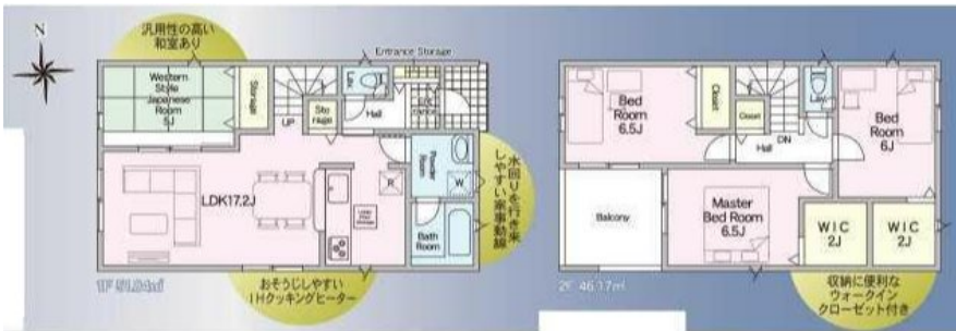
【間取り図】
