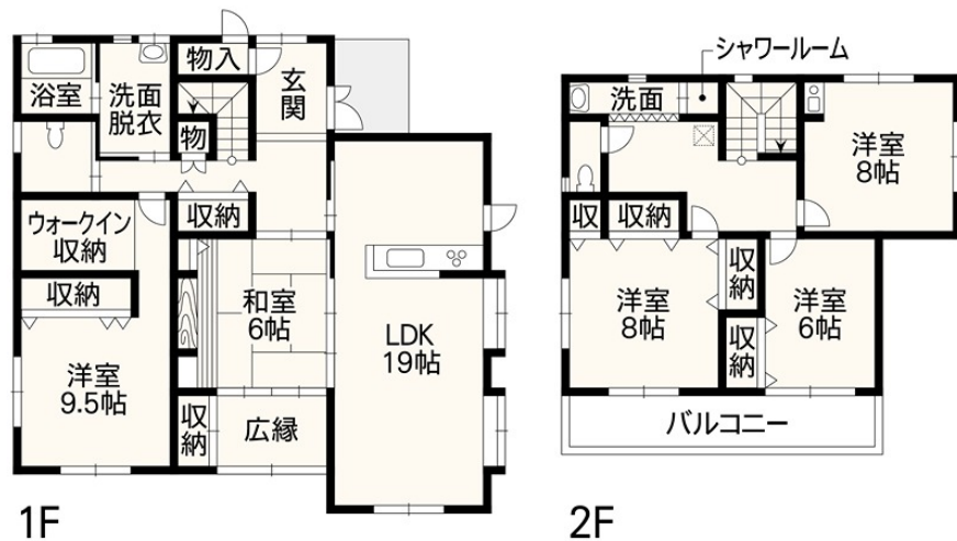
【間取り図】
