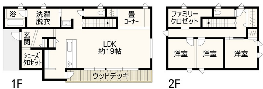
【間取り図】
